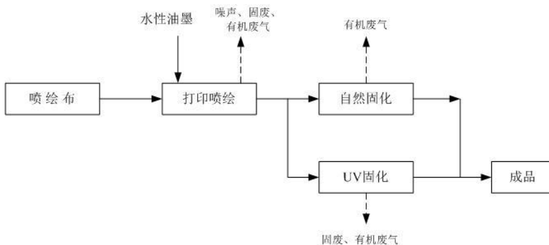
图5 工艺流程与污染产生环节
