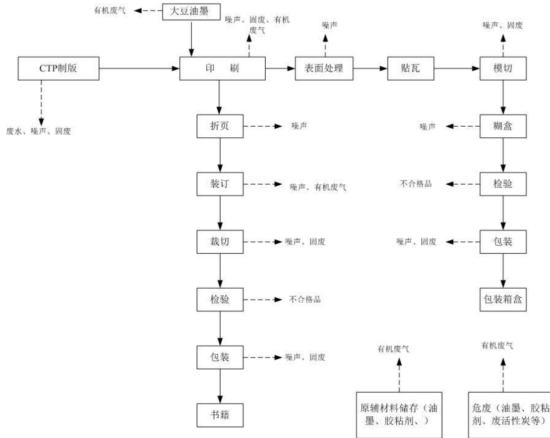
图 4 印刷纸制品生产工艺流程与污染产生环节
