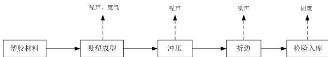
图3 广告门头吸塑字生产工艺流程与污染产生环节
