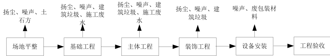
图2 施工期工艺流程与污染产生环节
